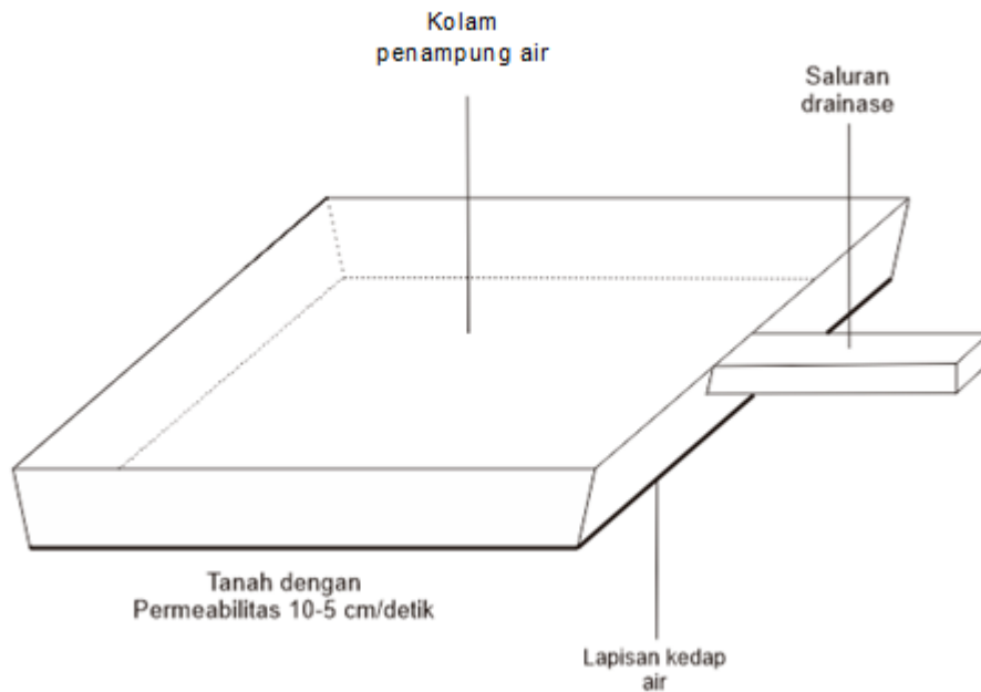
Gambar 6. Contoh Bak Penampung Tumpahan
